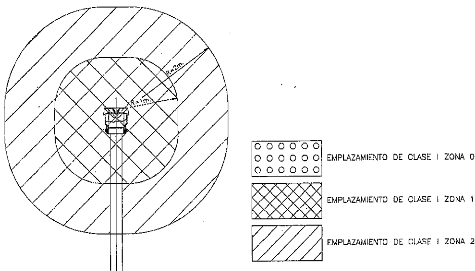
Fig. 5 – Detalle de clasificación del venteo.
