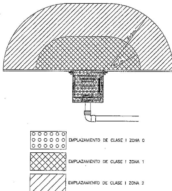
Fig. 4 – Detalle de clasificación de arqueta de descarga.
